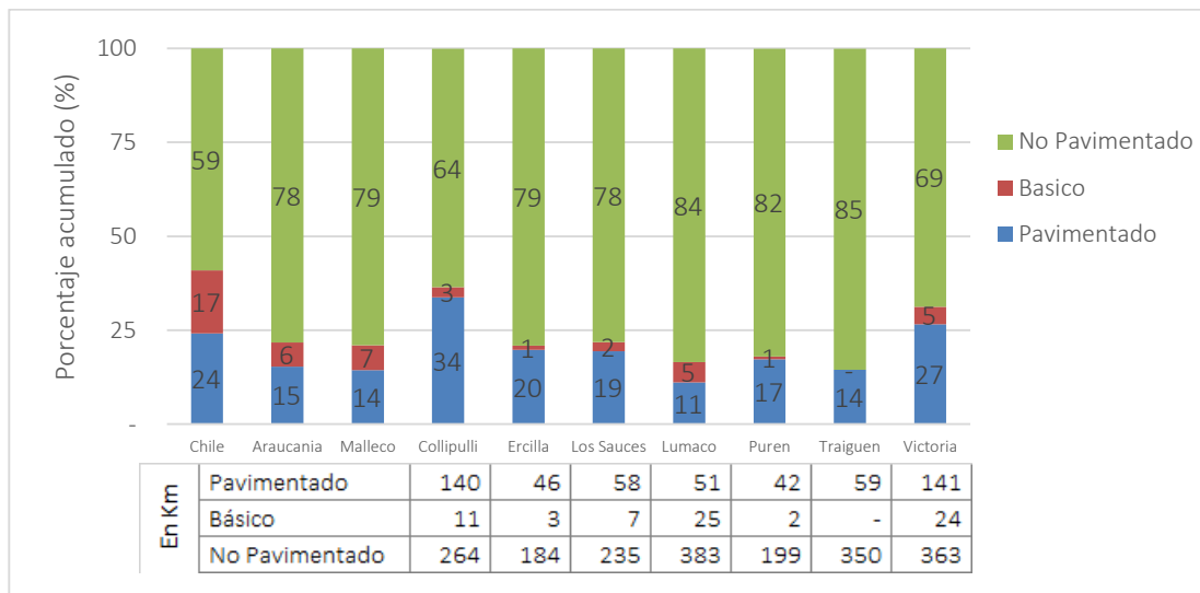
Gráfico 9: Red Vial según capa de rodadura
