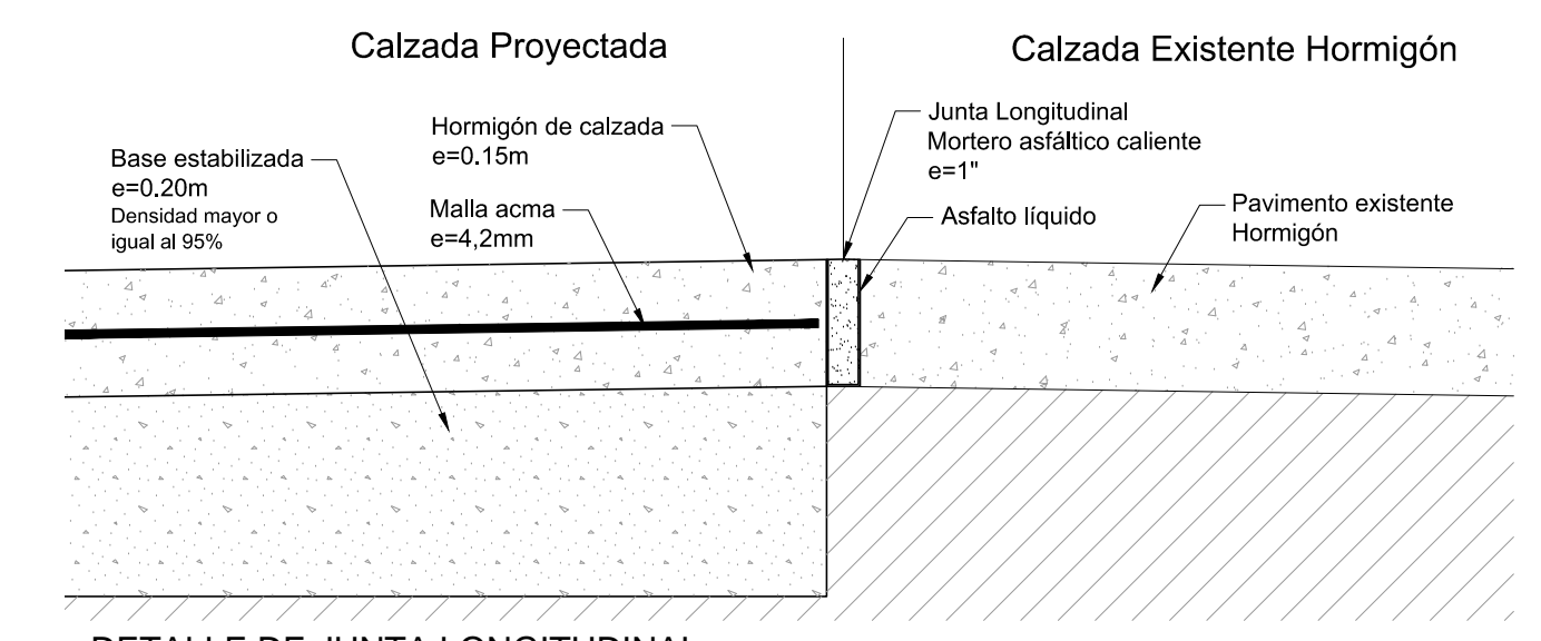
DETALLE DE JUNTA LONGITUDINAL Esc: 1/10
