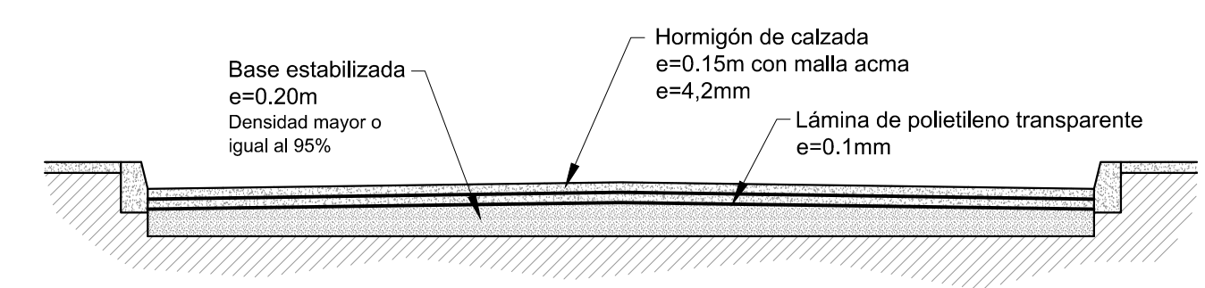
DETALLE CALZADA CALLE CARRERA Esc: 1/50
