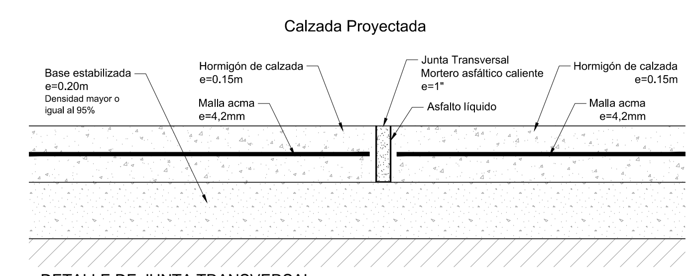
DETALLE DE JUNTA TRANSVERSAL Esc: 1/10
