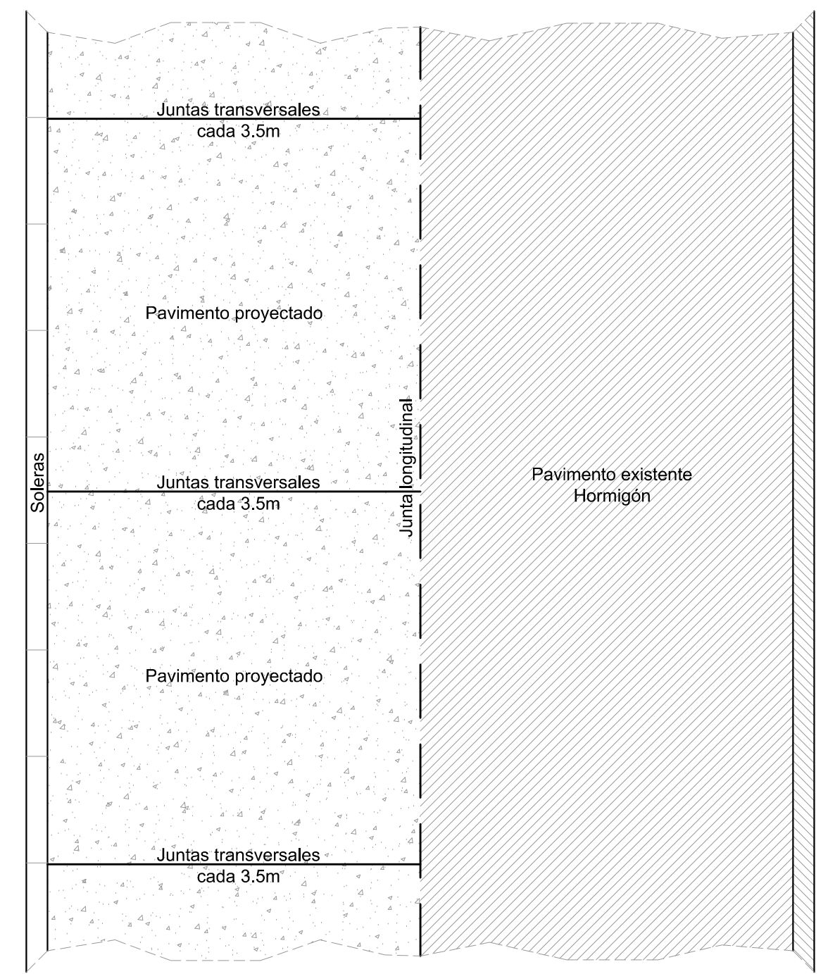
DETALLE DE JUNTAS CALZADA CALLE CARRERA Esc: 1/50
