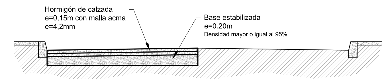
DETALLE CALZADA CALLE CARRERA Esc: 1/50
